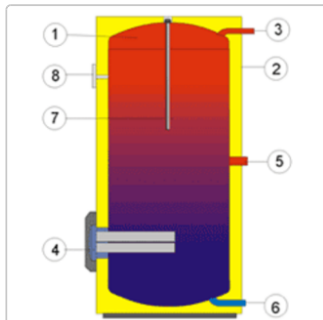
elektrische Warmwasserspeicher / Standspeicher
