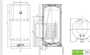
Oberer Aufhängung + unterer Aufhängung
