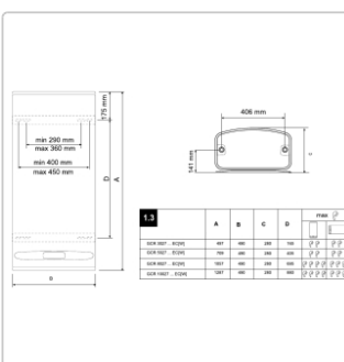
elektrische wandhängende Warmwasserspeicher - zur vertikalen oder horizontalen Aufhängung - sehr schlanke Ausführung - nur 28 cm tief - mit oder ohne WiFi
