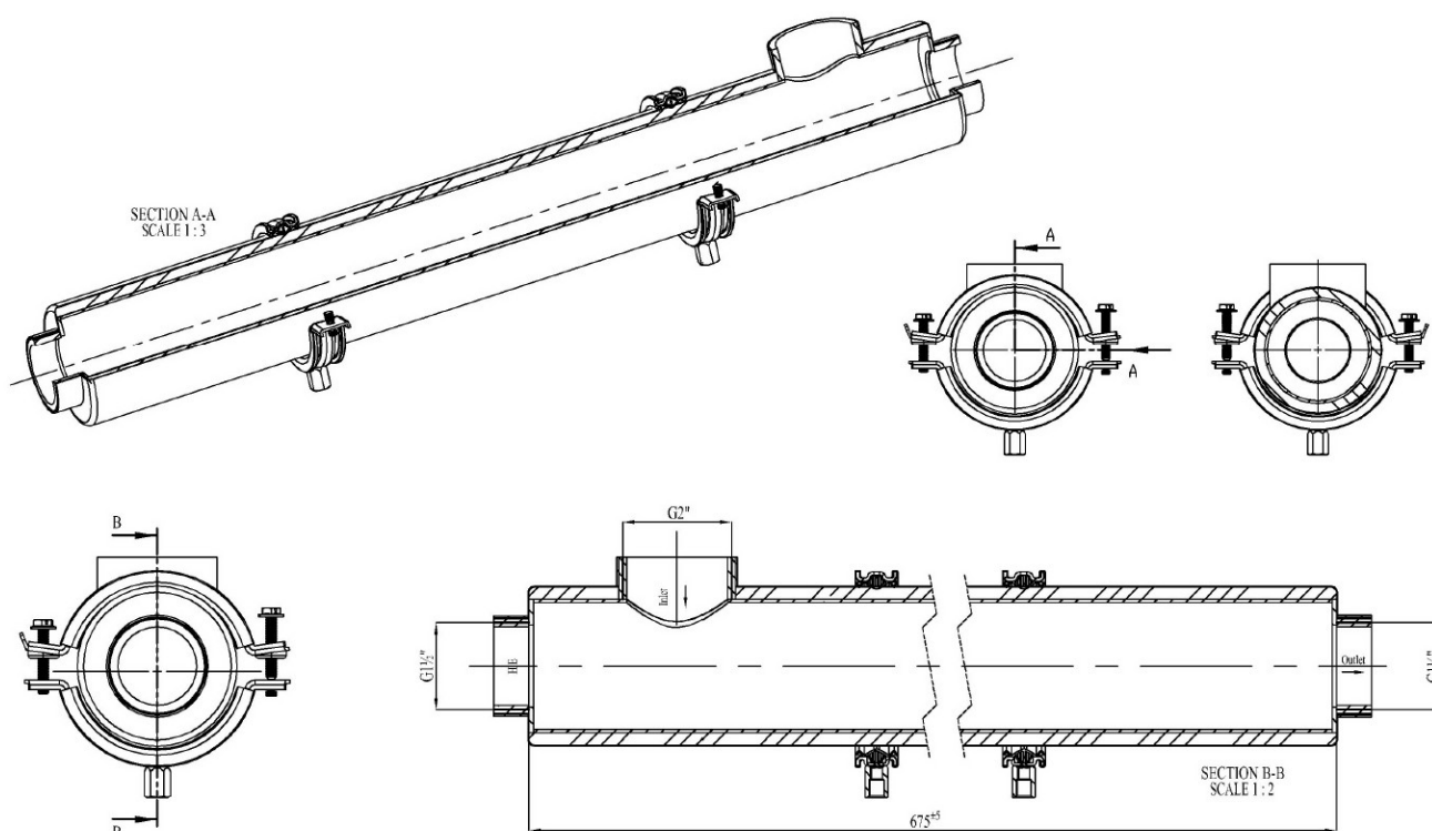
OPTIONALER ELEKTROHEIZSTAB
